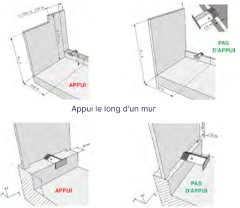
Exemples d'utilisation du gabarit pour identifier les appuis
